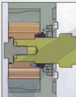
Sello mecánico simple
